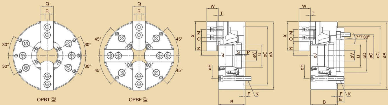
尺寸圖 > Dimensions
